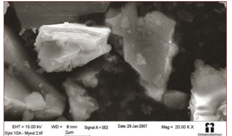
Rafeindasmásjármynd af óhreinindum af Miklubraut í Reykjavík. Öll korn á myndinni eru minni en 10µm og geta því auðveldlega þyrlast upp og breyst í svifryk. Orðið „ryk“ hljómar frekar sakleysislega. Sé horft á myndina koma frekar upp í hugann orð eins og bergflísar. Þarna má sjá hárfín oddhvöss korn sem óæskilegt er að anda að sér.
