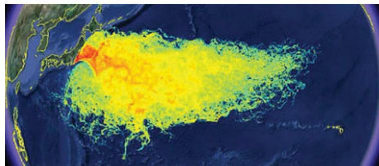
Geislaamengun í Kyrrahafi frá kjarnorkuverinu í Fukushima.
