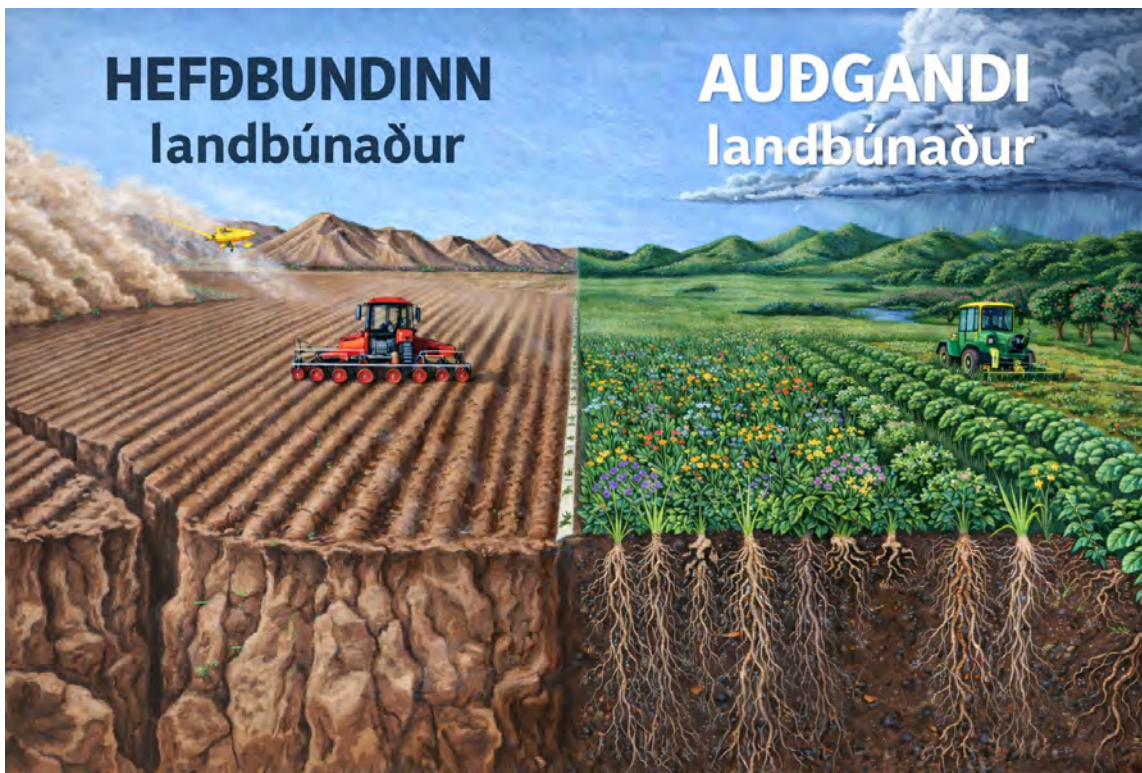
Skýringarmynd sem sýnir hvernig jarðvegsbygging og rótarkerfi hafa áhrif á vatnsbúskap, lífríki og seiglu landbúnaðar.
