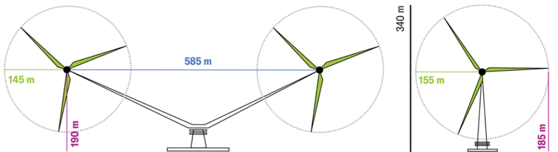
T.v. er fyrirhuguð 50 MW tveggja snúningsása vindmylla Ming Yang Smart Energy. T.h. er núverandi stærsta vindmylla heims. Teikning / Ming Yang Smart Energy
