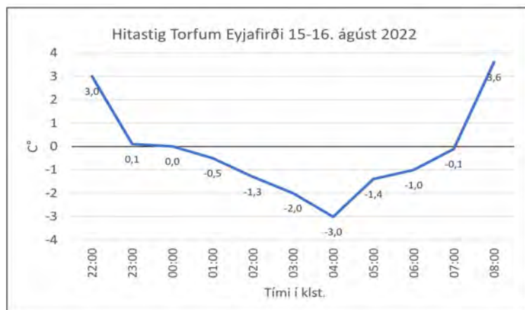
3. mynd. Hitastig á Torfum 15.-16. ágúst 2022.
