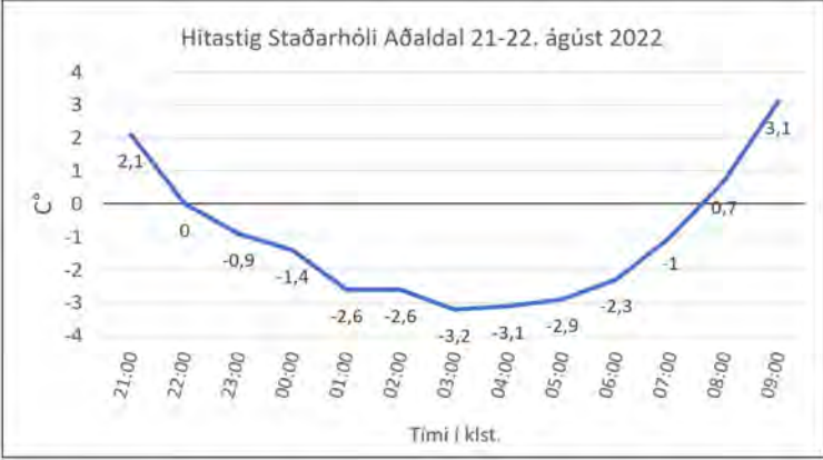
8. mynd. Hitastig á Staðarhóli í Aðaldal 21.–22. ágúst 2022.
