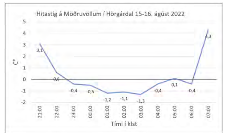
5. mynd. Hitastig á Möðruvöllum 15.-16. ágúst 2022.
