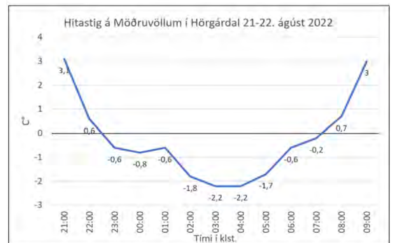
6. mynd. Hitastig á Möðruvöllum 21.-22. ágúst 2022.
