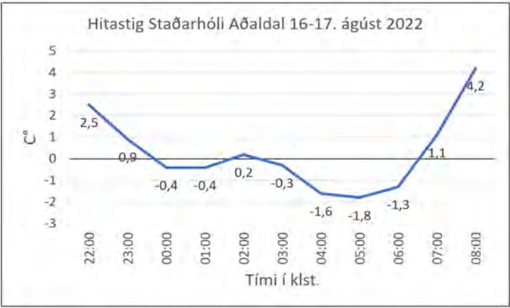
7. mynd. Hitastig á Staðarhóli Aðaldal 16.–17. ágúst 2022.
