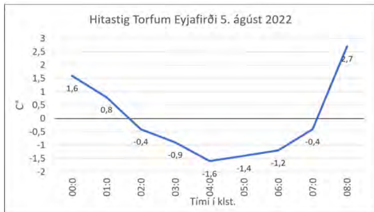
2. mynd. Hitastig á Torfum 5. ágúst 2022.
