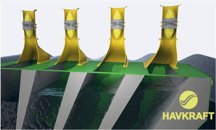
Haf-Afl ehf. hyggst setja upp fljótandi ölduorkustöðvar, 100 MW, sem miðar að raforkusjálfbærni Vestmannaeyja árið 2030. H-WEC OWC ölduorkubreytir samstarfsfyrirtækisins Havkraft. Mynd / Aðsend
