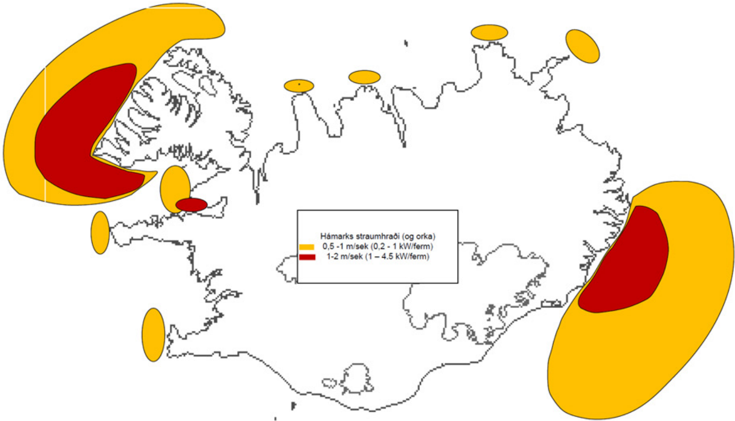
Nýtanleg sjávarorka við Ísland. Hámarks straumhraði (og orka). Gult: 0,5-1 m/sek (0,2-1 kW/ferm). Rautt: 1-2 m/sek (1-4,5 kW/ferm.). Kort / Skýrsla Valorku
