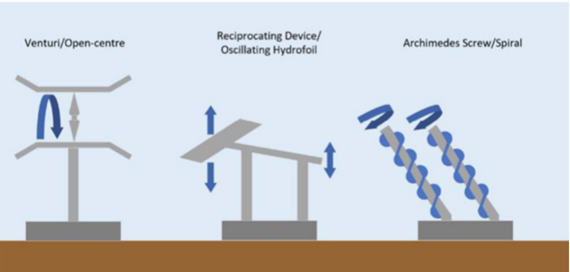
Tækni til að beisla orku sjávarstrauma. Efri röð frá vinstri: Láréttur ás-fastur. Láréttur ás-fljótandi. Lóðréttur ás. Sjávarfallaflugdreki. Neðri röð frá vinstri: Venturi-opin-miðja. Gagnkvæmnistæki/sveifluvatnsflaumur. Arkimedesarskrúfa/spirall. Mynd / Skýrsla Valorku.
