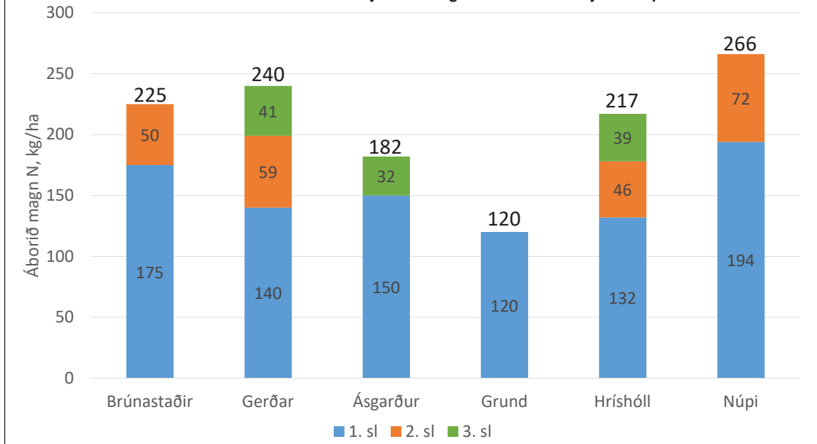
MYND 3: Áborið köfnunarefni með búfjáráburði og tilbúnum áburði hjá öllum þátttakendum
