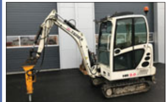
Terex HR 2.0 smágrafa. Árgerð 2006. 3.150 vinnust. 3 skóflur og fleygur.
