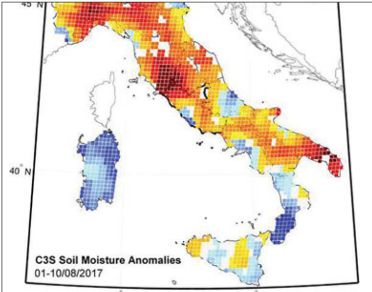
Staða rakamælinga í jarðvegi á Ítalíu 10. ágúst 2017.
