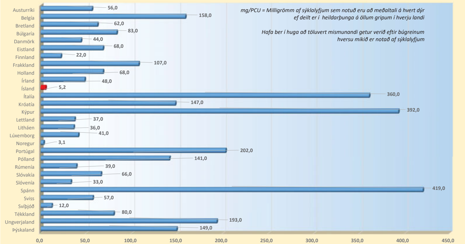
Notkun sýklalyfja handa búfé í 29 Evrópulöndum árið 2014, mælt í mg/PCU.
