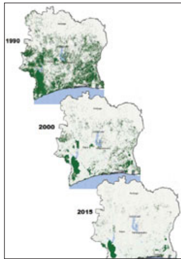
Skógareyðing á Fílabeinsströnd Afríku frá 1990 til 2015.
