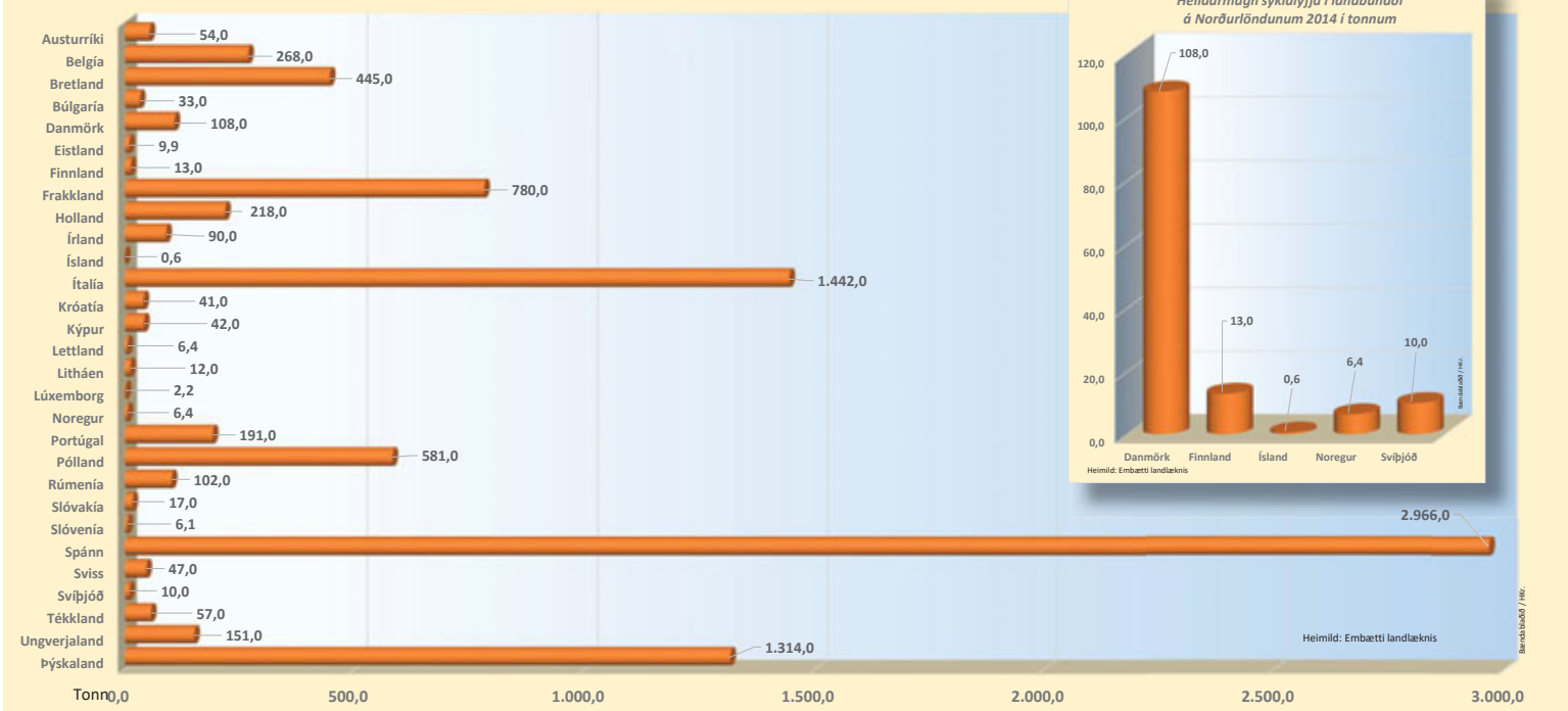
Heildarmagn sýklalyfja í landbúnaði í 29 Evrópulöndum 2014 í tonnum
