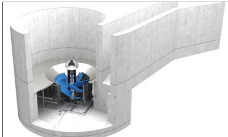
Í þessari hönnun er hluti lækjarins látinn renna í gegnum þetta mannvirki sem myndar vatnshvirfil líkt og þegar tappi er tekin úr baðkari. Það gefur stóruorku orku þótt fallhæðin sé sáralítill.
