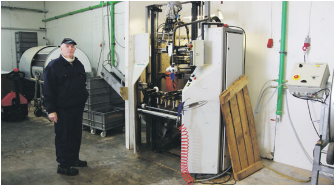
Ásgeir við danska pelsunartækið sem leysti af fjóra fláningsmenn á búinu. Í vélinni flær Eistlendingurinn Andrus um 600 minka á dag og er þá aðeins um 15 sekúndur með hvert dýr.
