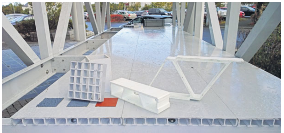
Hægt er að fá margvíslega prófíla úr FRP-efni frá Fiberline Composites A/S í Danmörku.
