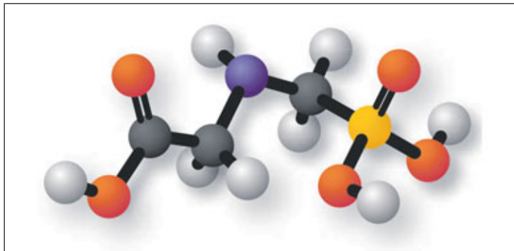
Líkan af uppbyggingu glýfósats.
