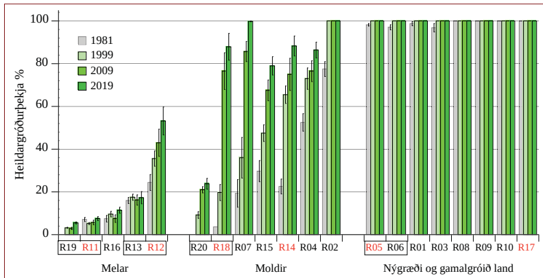
2. mynd. Heildargróðurþekja í reitum við Heygil á Hrunamannaafreitti 1981–2019. Friðaðir reitir eru merktir með rauðum lit. Þeir reitir sem eru nokkurn veginn sambærilegir eru tengdir með ferhyrningum. Innan hvers reits var mælt í 10 eins fermetra smáreitum. Lóðrétt strík tákna staðalskekkju.
