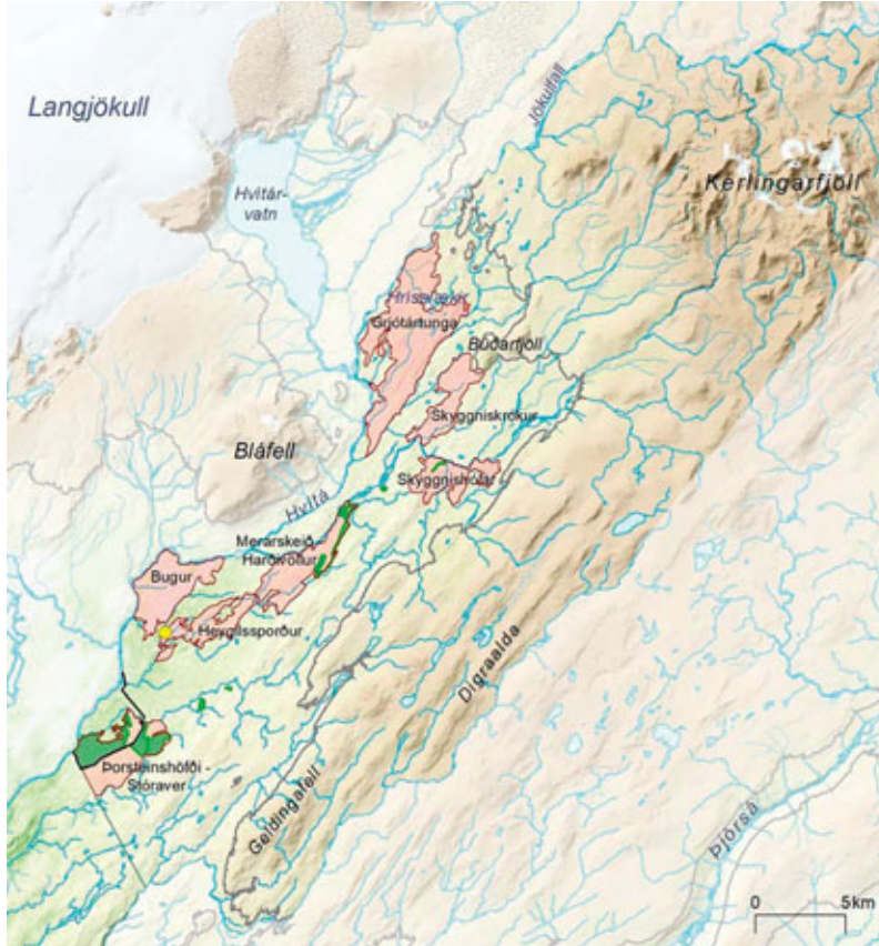
1. mynd. Hrunamannaafreittur, sem er um 1000 km 2 að flatarmáli, er á suðvesturhálendinu austan Hvítár. Hæð yfir sjó er frá um 250 m suðvestast í afrétti upp í 1488 m í Kerlingarfjöllum; 500 m hæðarlina er sýnd með gráum lit. Landgræðslugirðing suðvestast í afrétti er merkt með svartri línu. Helstu rofsvæði eru sýnd í rauðum lit en uppgræðslusvæði græn. Rannsóknasvæðið við Heygil er merkt sem gulur punktur.
